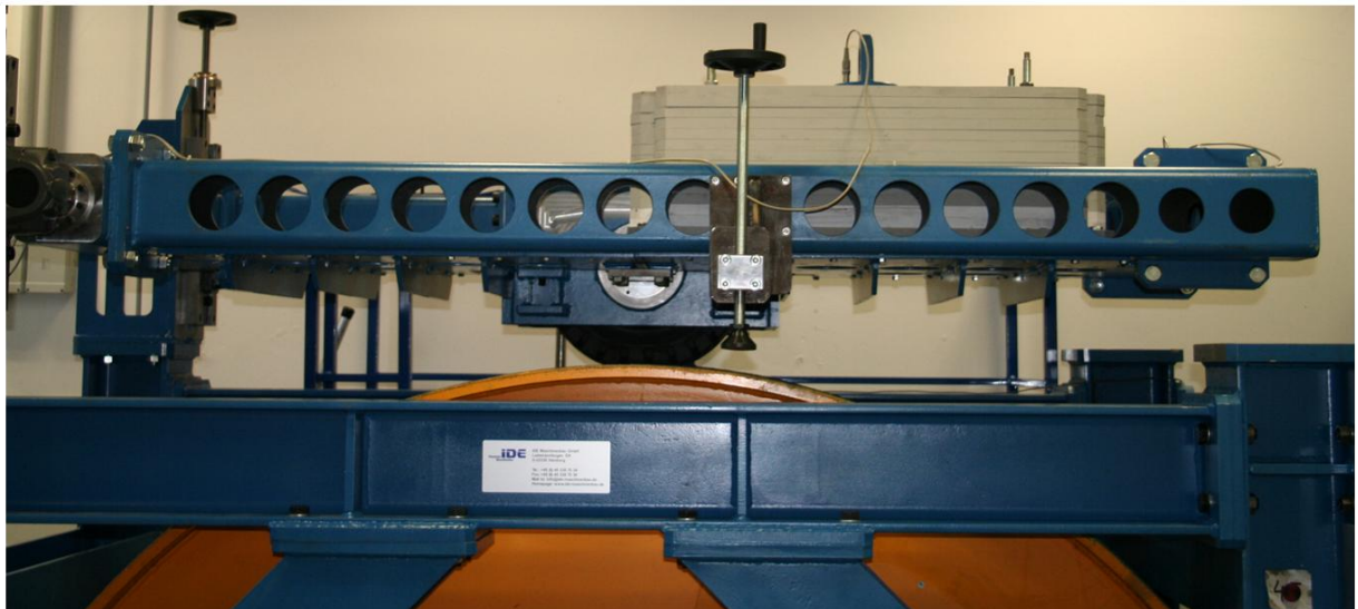
Abbildung 2: Versuche am Trommelprüfstand
